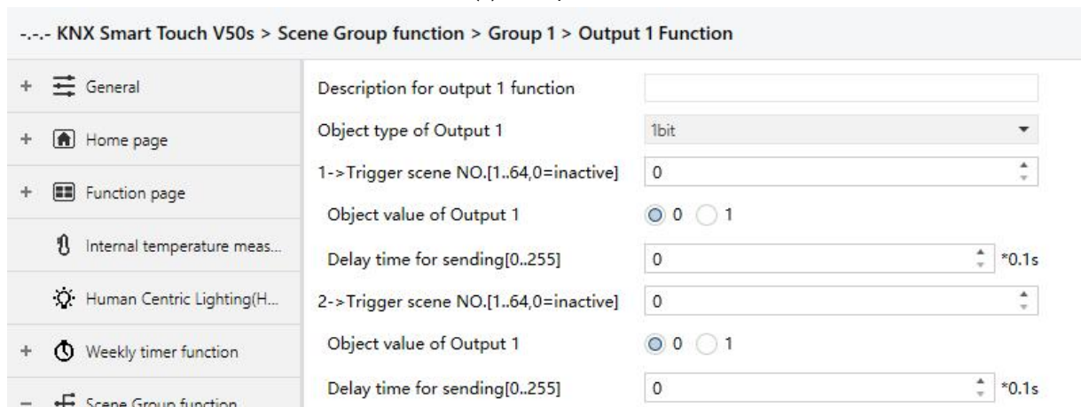
图 5.7(3) “Output y Function” 参数设置界面
