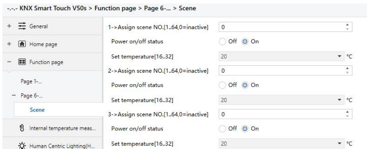
图 5.3.7.1 “Scene” 参数设置界面
