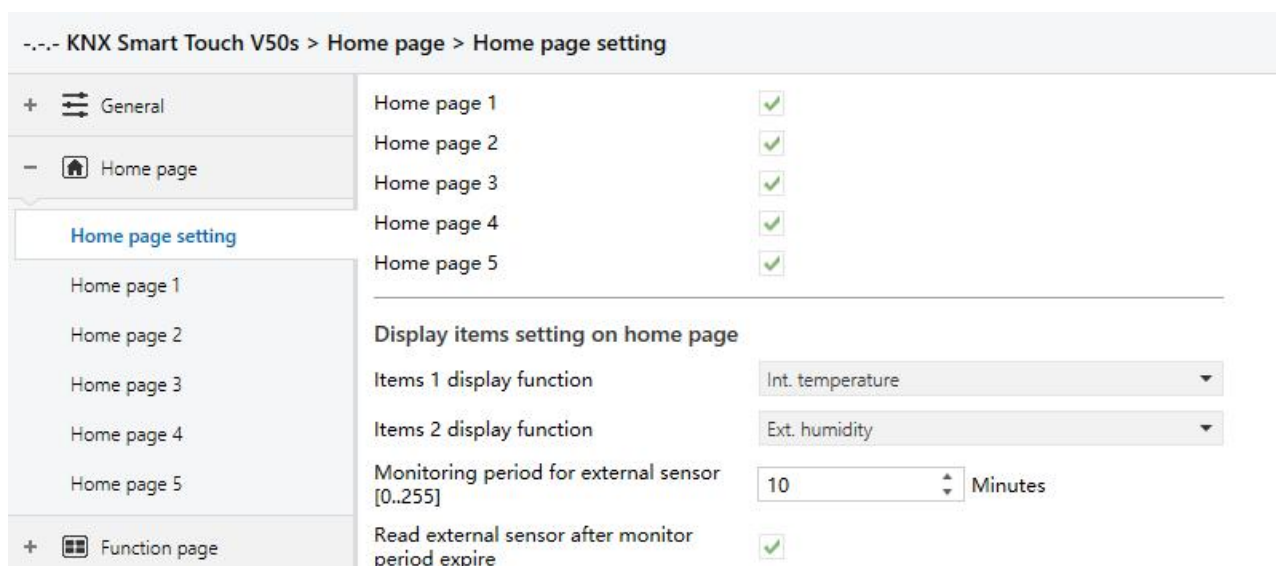
图 5.2.1 “Home page setting” 参数设置界面
