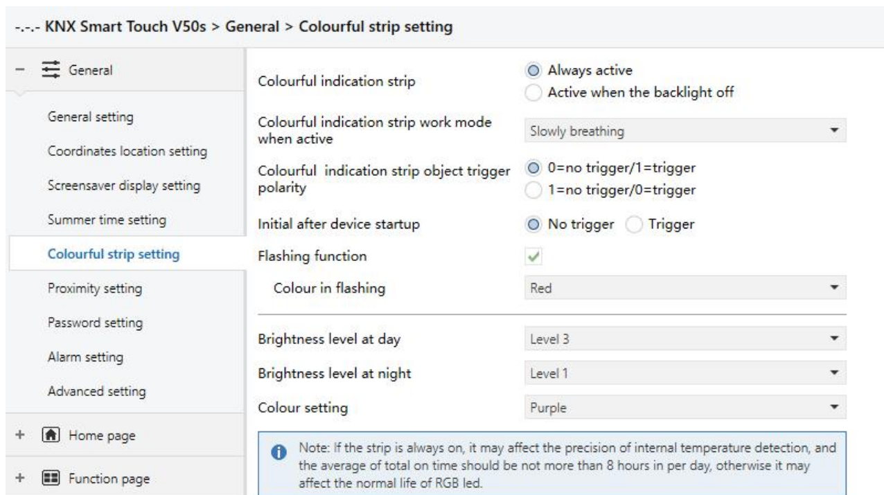
图 5.1.5 “Colourful strip setting” 参数设置界面
