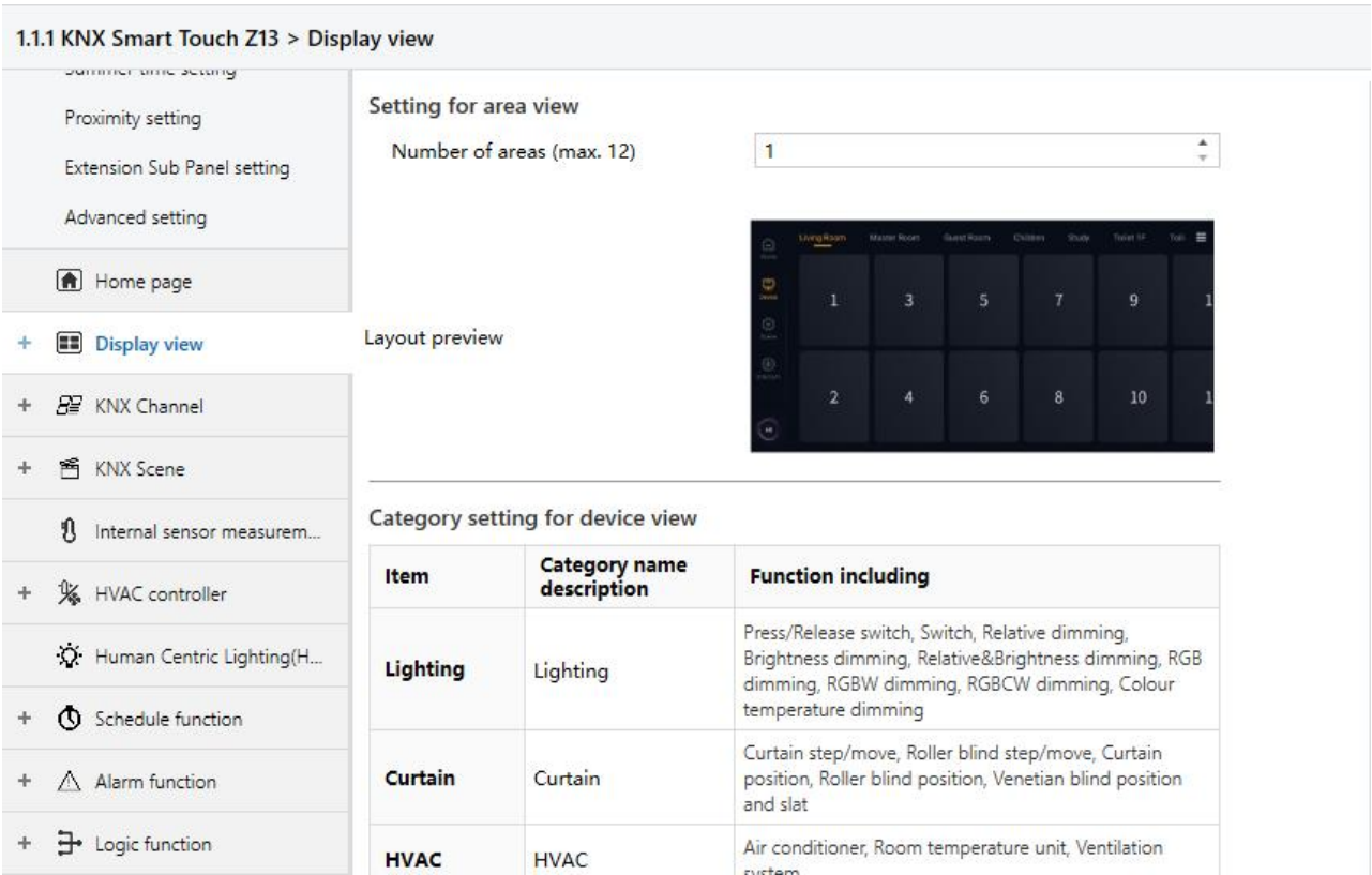
图 5.10 “Display view”参数设置界面
