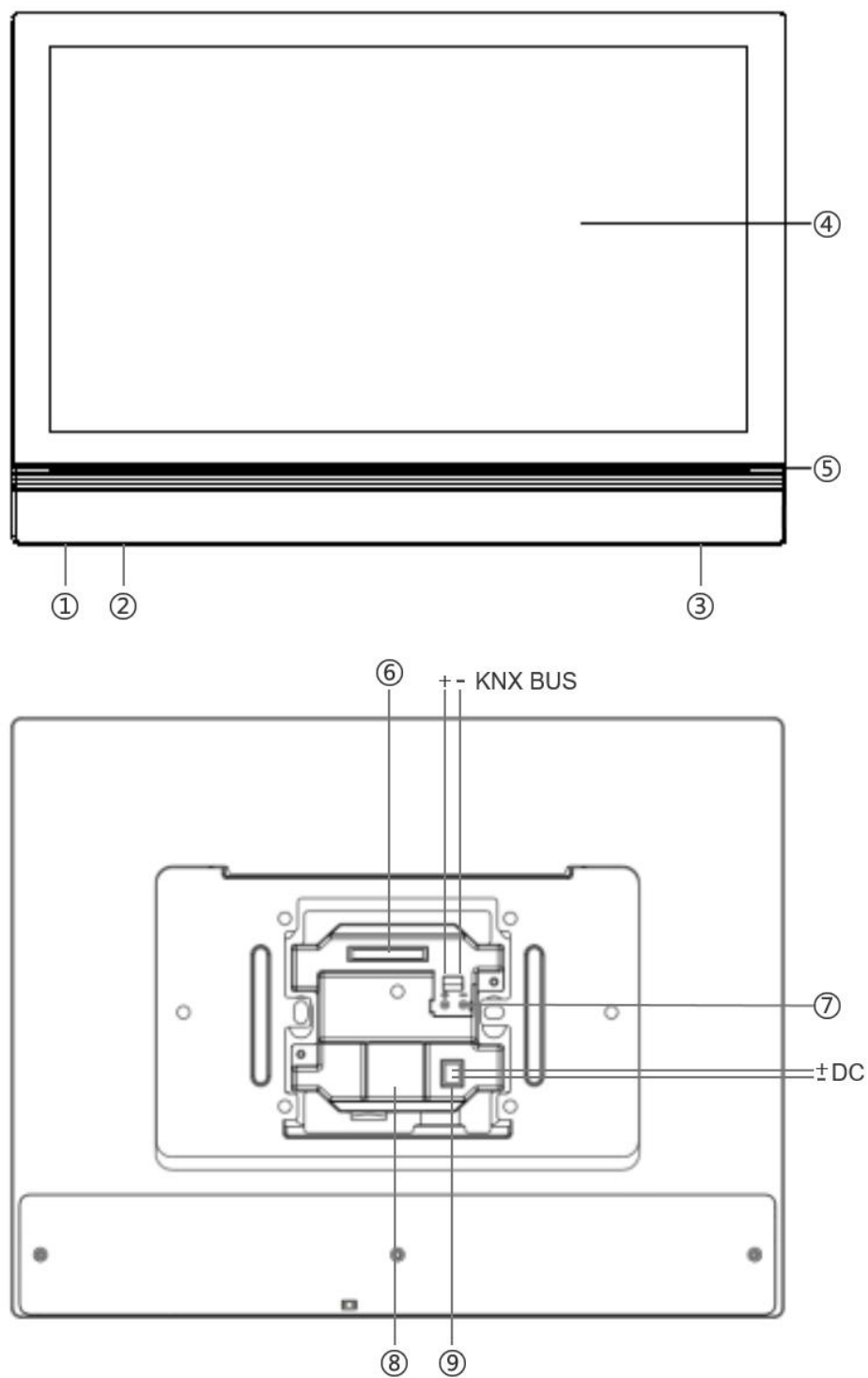
图 3.1 KNX 智能屏 Z10 接线图
