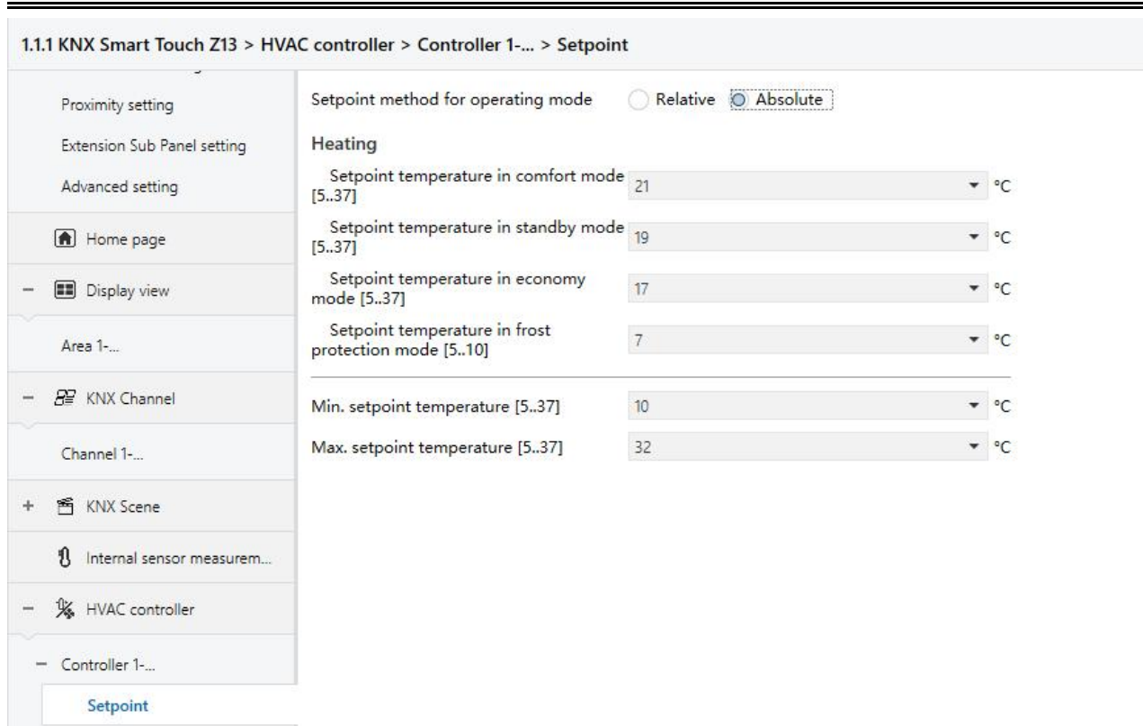
图 5.3.1.1 “Setpoint” 参数设置界面
