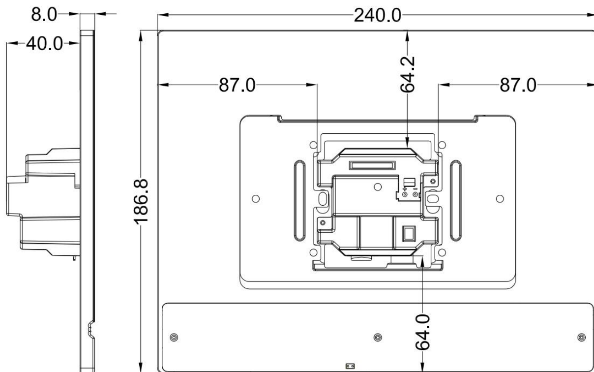
图 3.1 KNX 智能屏 Z10 尺寸图
