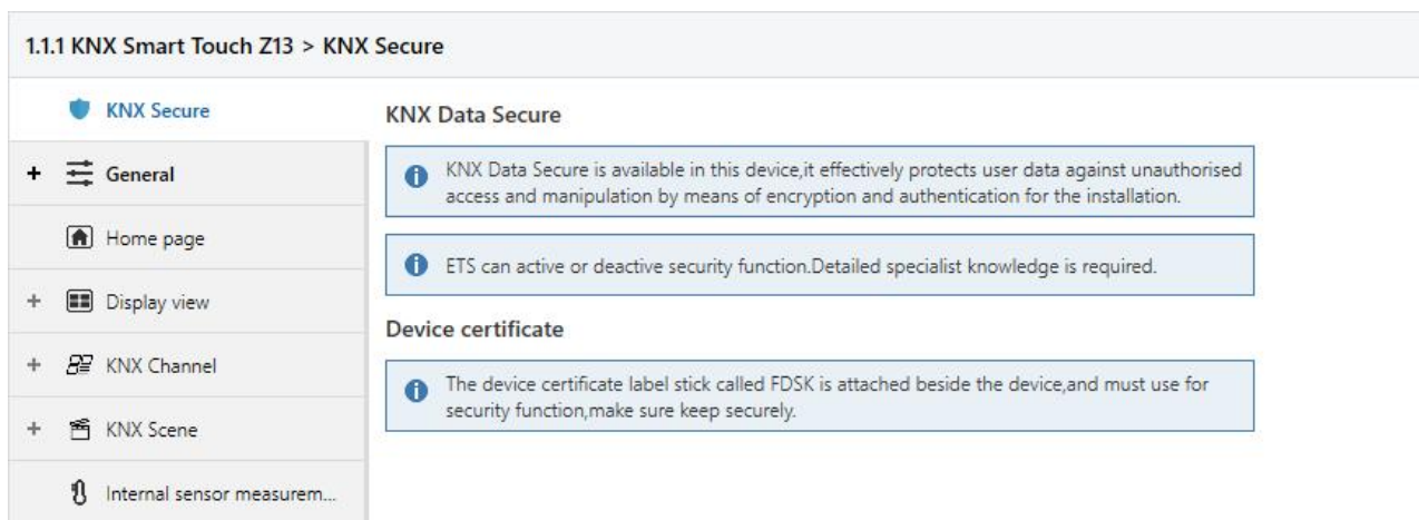
图 5.1 (1) “KNX Secure” 参数界面
