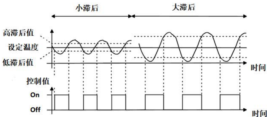
图 5.3.1.2(2) 两点控制方式下滞后对控制值开关动作的影响 (加热)
