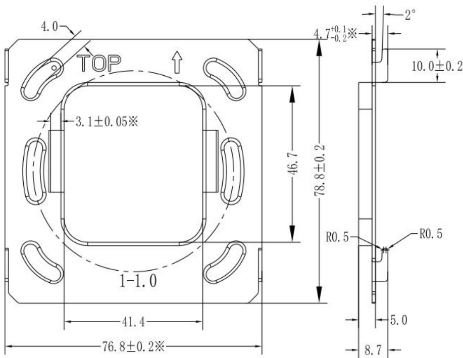
图 3.1.5 CHTF-4.0/15.3.2x 挂板尺寸
