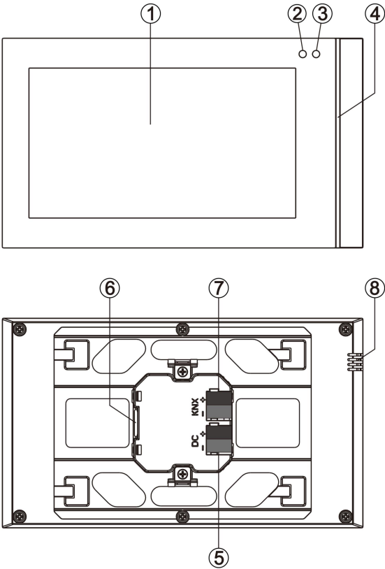
图 3.2.3 CHTF-5.0/15.4.2x 接线图
