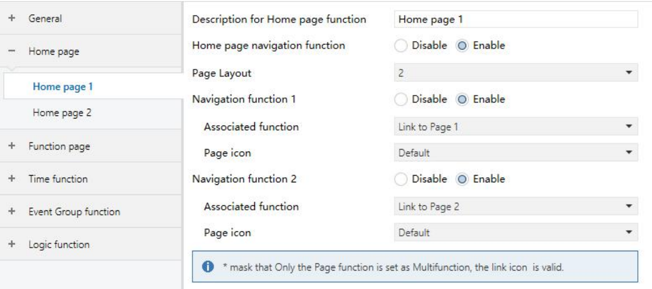
图 5.2.1 “Home Page x” 参数设置界面
