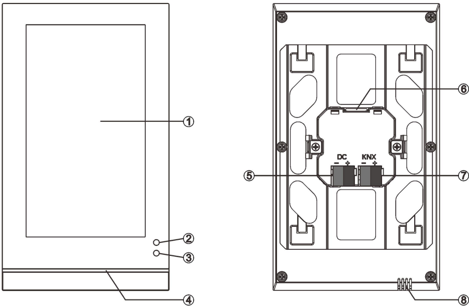
图 3.2.2 CHTF-5.0/15.3.2x 接线图
